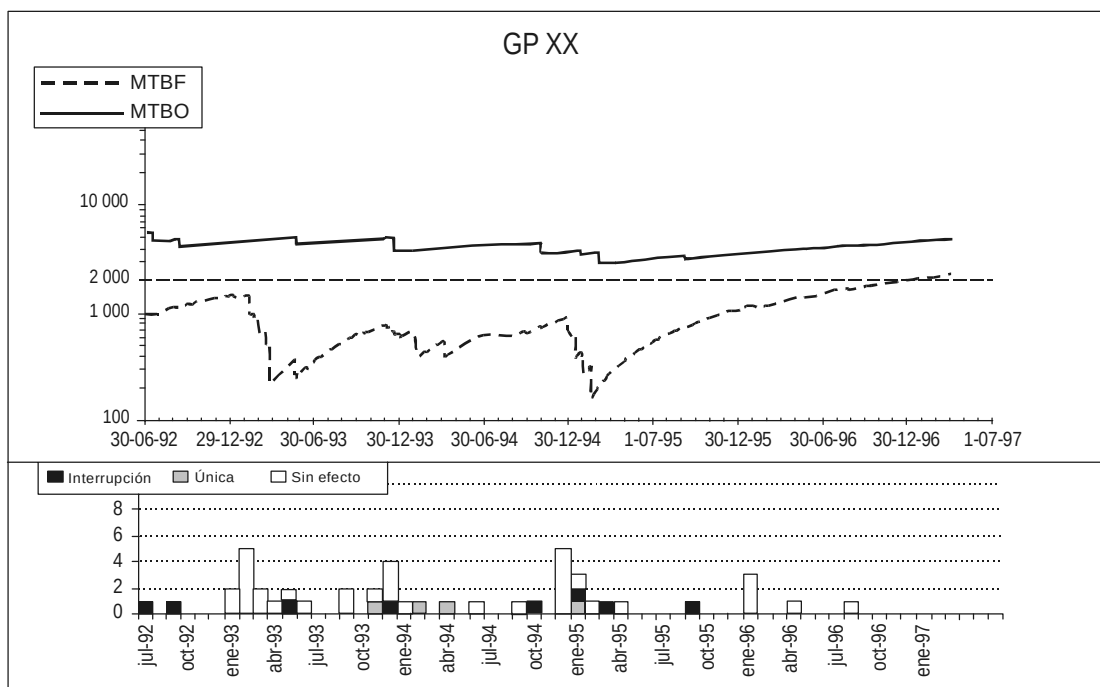
Figura C-12B. Ejemplo de registro de interrupciones de una trayectoria de planeo
