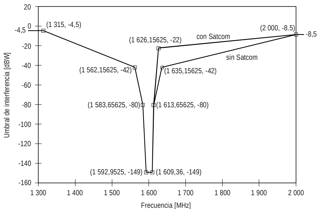
Figura B-16. Umbral de interferencia CW para receptores GLONASS utilizados en aproximaciones de precisión
