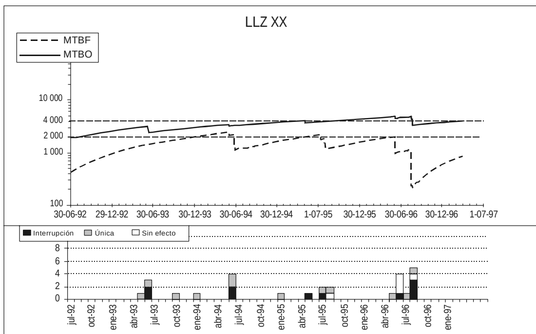
Figura C-12A. Ejemplo de registro de interrupciones de un localizador
