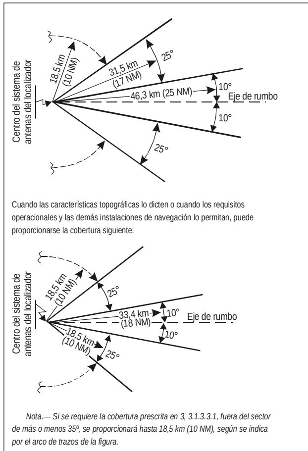
Figura C-7. Cobertura del localizador en azimut
