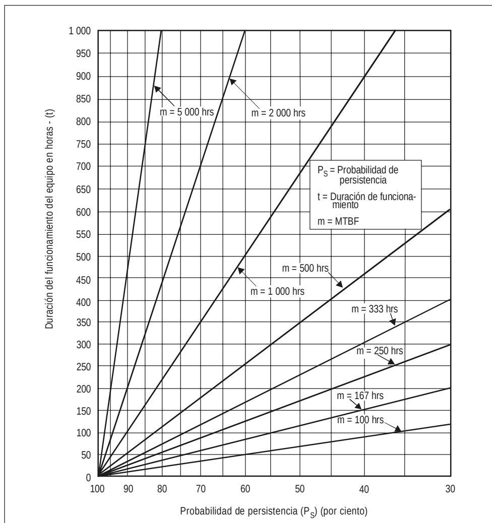
Figura F-1. Gráfico de P_s = 100 e^{-t/m}
