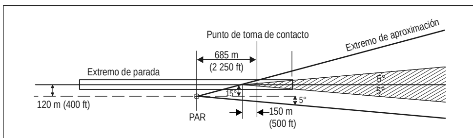
Figura C-16. Retroceso mínimo del PAR respecto al punto de toma de contacto, para una desviación de 120 m (400 ft), cuando esté alineado para explorar 5 y 15^\circ respecto al QDR de la pista
