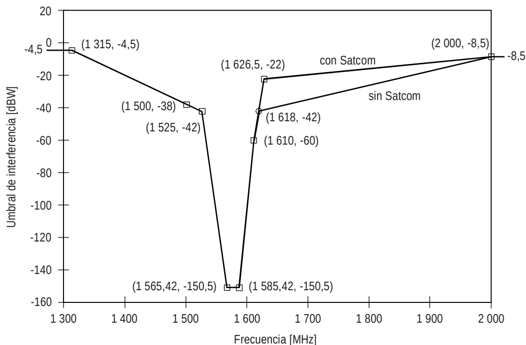
Figura B-15. Umbral de interferencia CW para receptores GPS y SBAS utilizados en aproximaciones de precisión
